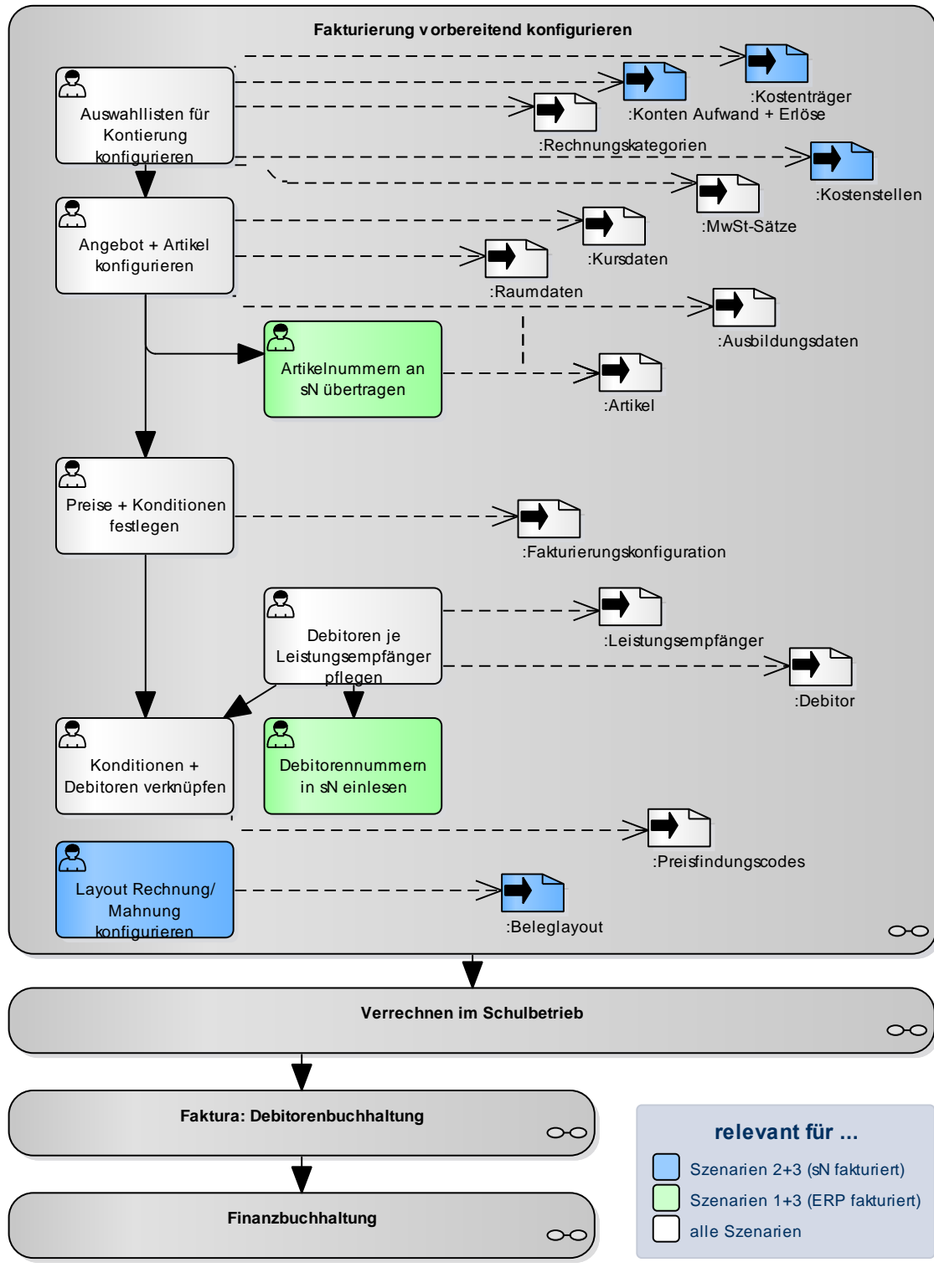
Abbildung 3 : Fakturierung Konfiguration
